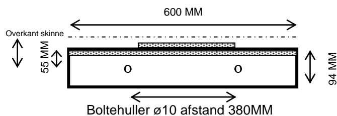
Modulkasse med mål set fra enden
