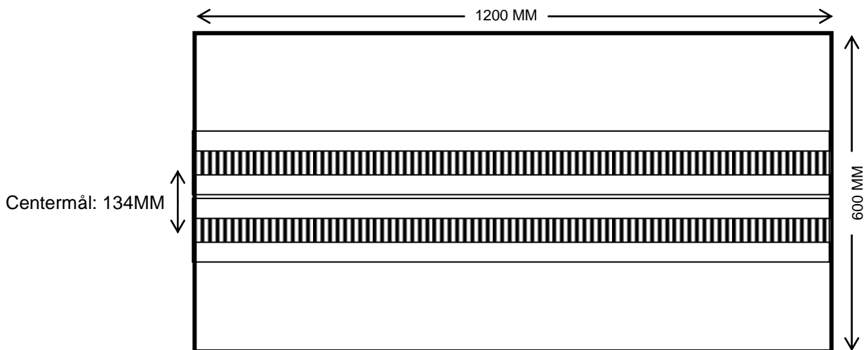
Modulkasse med mål set oven fra
